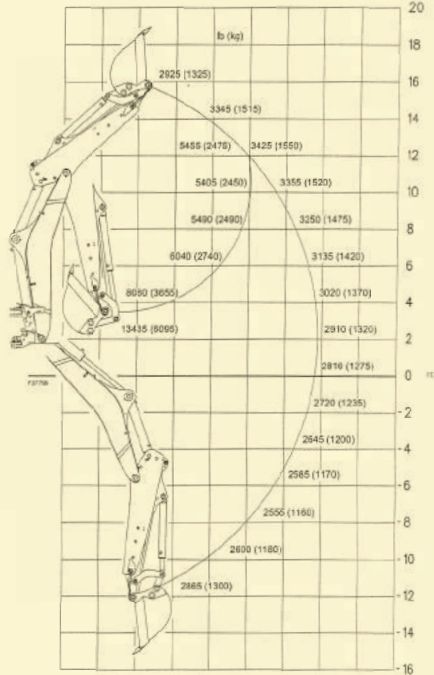
BRAZO CON AGUILÓN EXTENSIBLE HED, CORTO RETRAÍDO Y CUCHARA HD 610 mm (156 kg) / Cuchara de Cargadora 6 x 1
